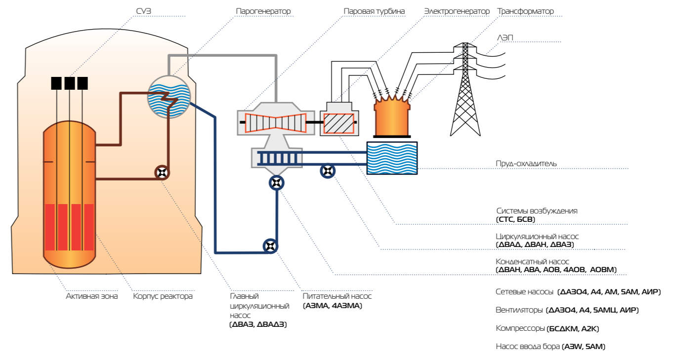
Схема расположения электродвигателей Русэлпром на атомной станции
